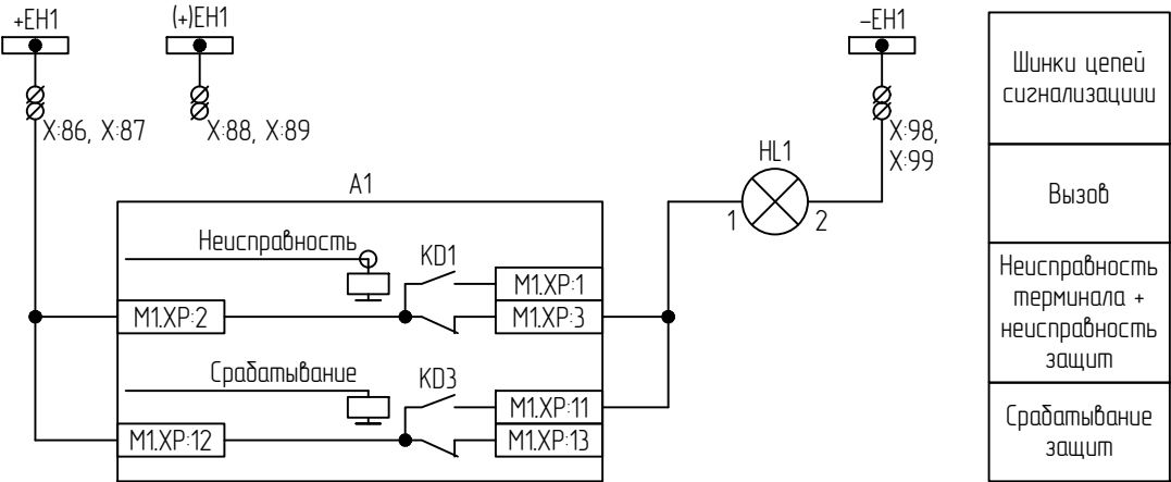
Цепи РАС
